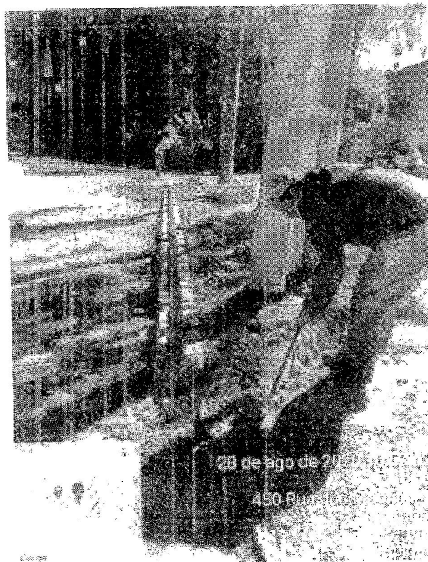
4 – Assentamento de meio fio na Rua dos Gerânios
