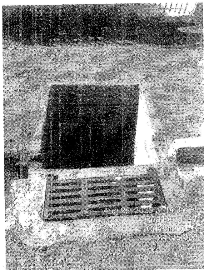
7 – Acabamentos nos dispositivos de drenagem
